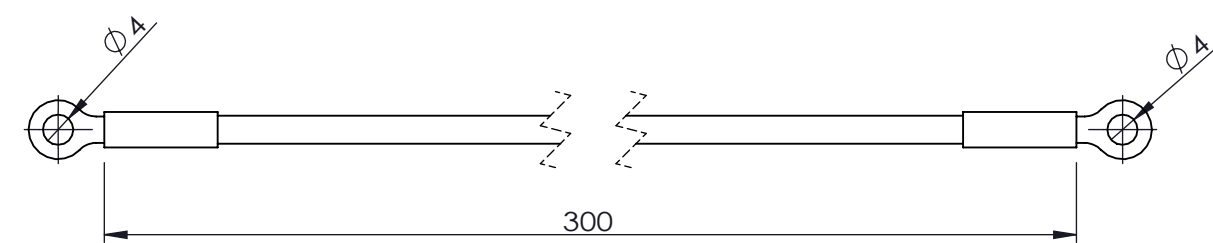
Earth Cable 1:1
